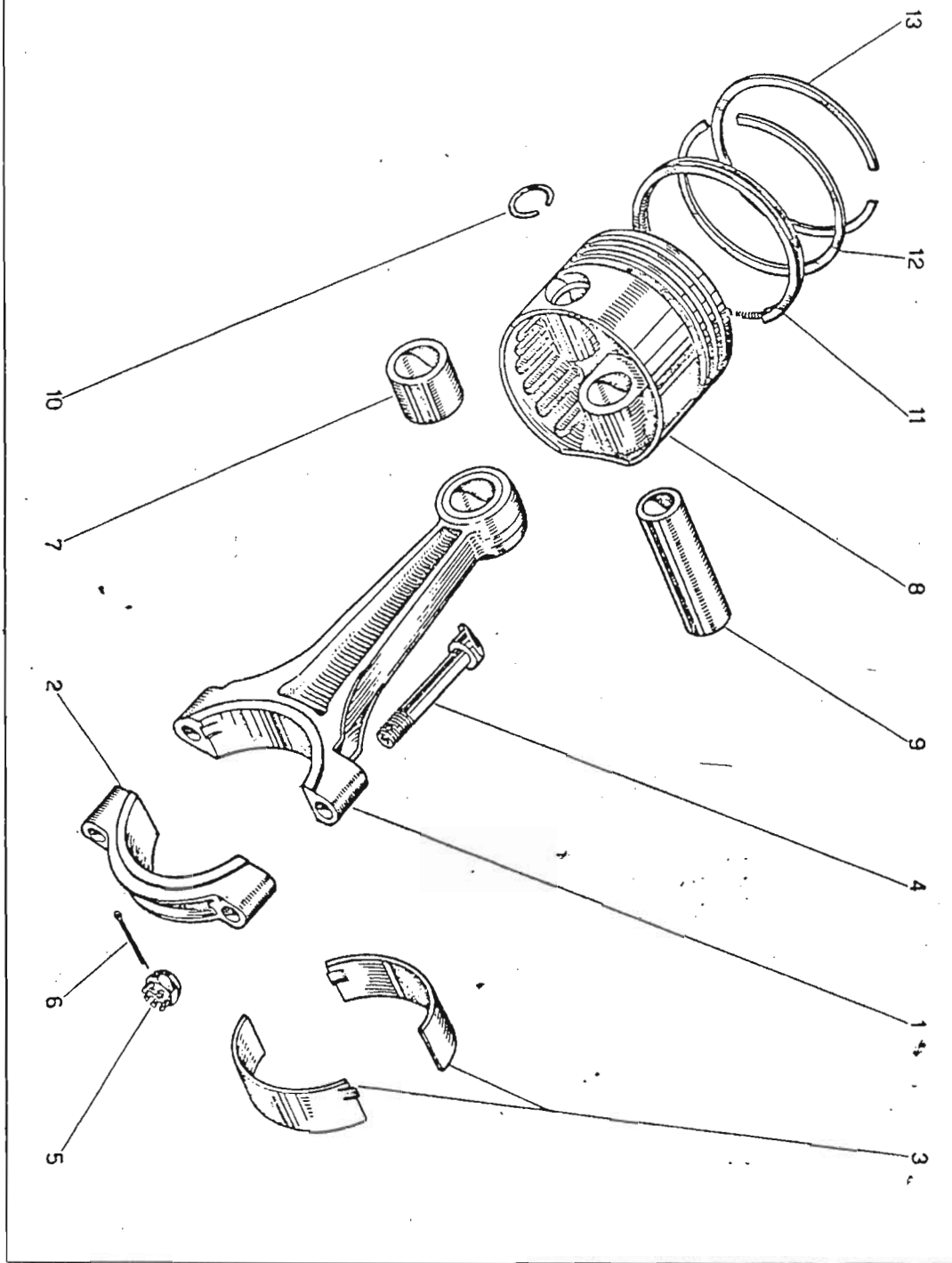
TAV. 4 - BIELLE E PISTONI
